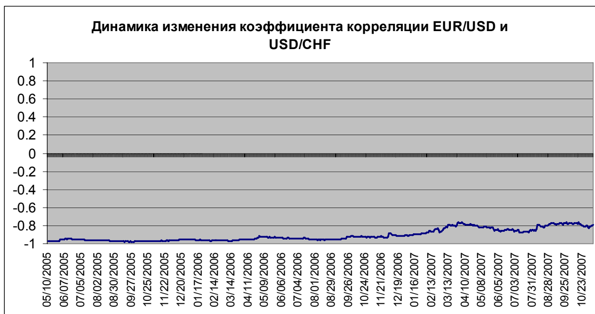
Рис. 31. График динамики изменения коэффициента корреляции , рассчитанный по дневным логарифмическим доходностям курсов валют EUR/USD и USD/CHF с временным интервалом 3 месяца с шагом 1 день. Валюты показывают сильную отрицательную взаимосвязь (при росте одной валюты другая падает).
