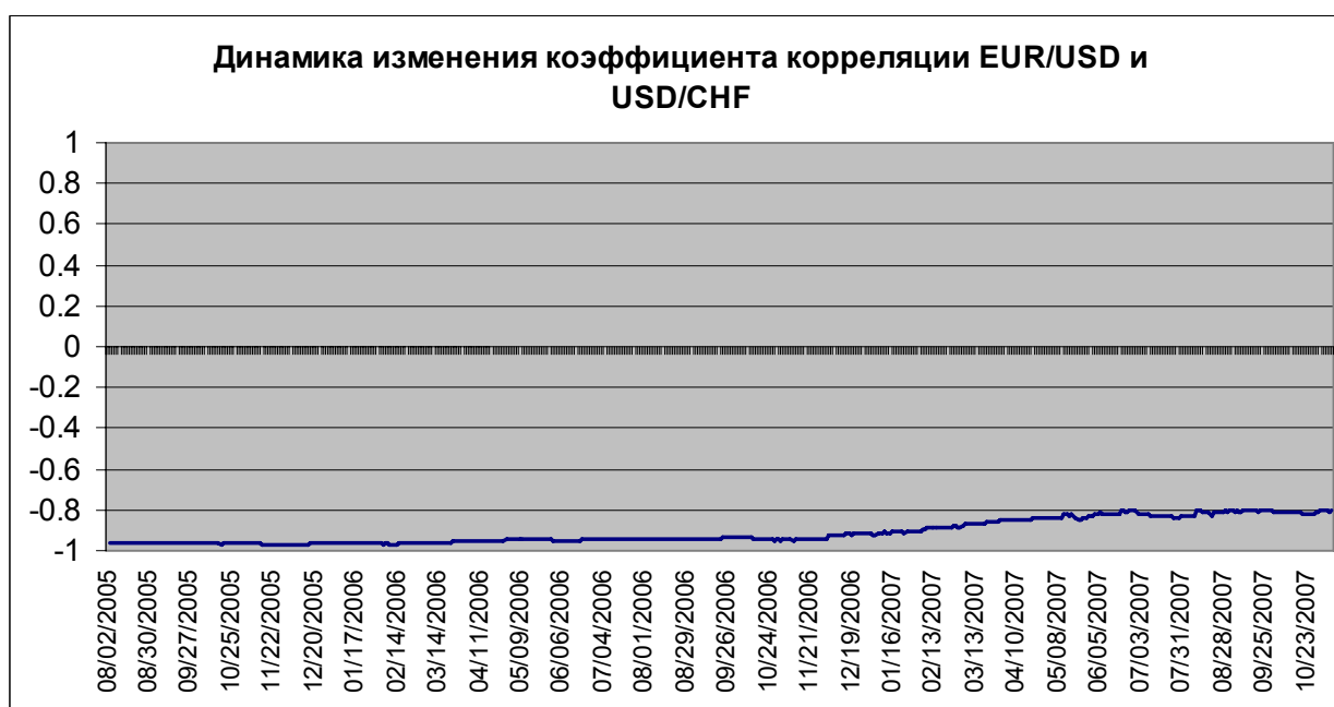
Рис. 32. График динамики изменения коэффициента корреляции , рассчитанный по дневным логарифмическим доходностям курсов валют EUR/USD и USD/CHF с временным интервалом 6 месяцев с шагом 1 день. Валюты показывают сильную отрицательную взаимосвязь (при росте одной валюты другая падает).
