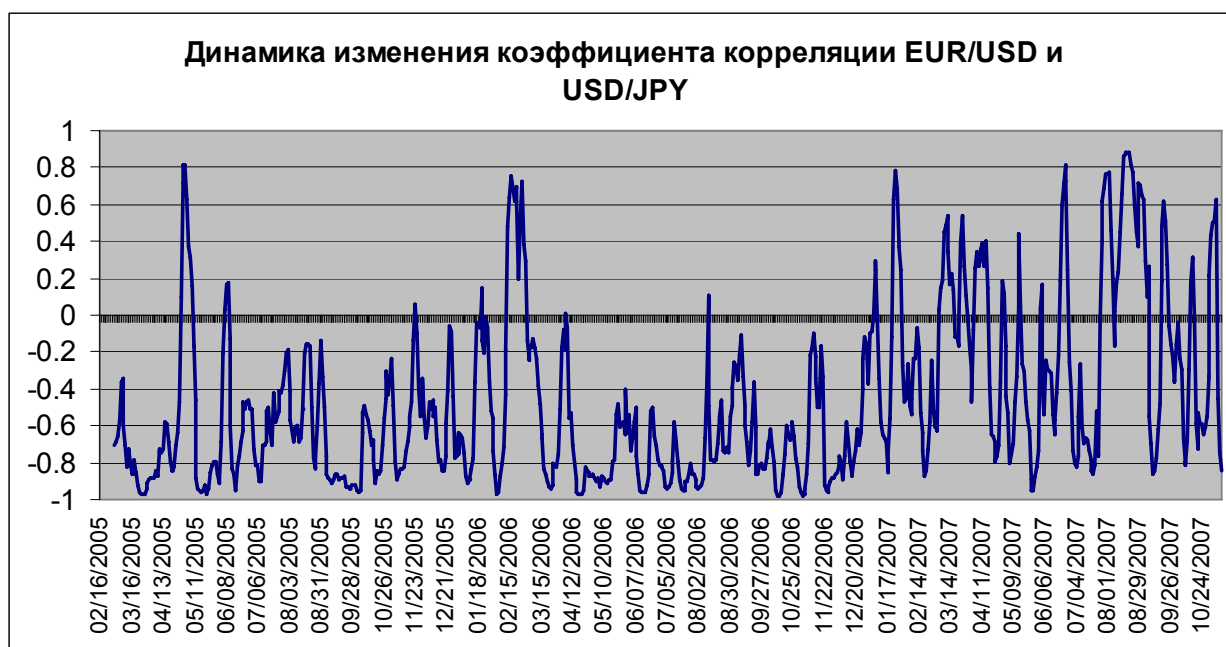
Рис. 17. График динамики изменения коэффициента корреляции по дневным ценам закрытия курсов валют EUR/USD и USD/JPY с временным интервалом 2 недели с шагом 1 день. Ситуация аналогична предыдущему графику.
