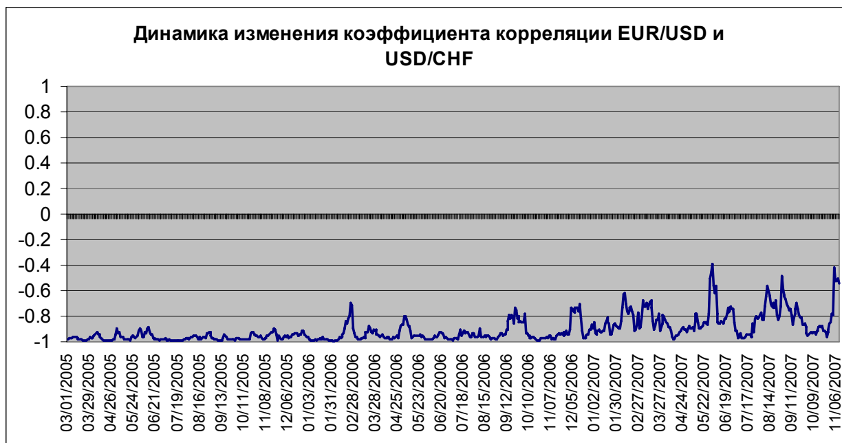
Рис. 29. График динамики изменения коэффициента корреляции , рассчитанный по дневным логарифмическим доходностям курсов валют EUR/USD и USD/CHF с временным интервалом 2 недели с шагом 1 день. Валюты показывают сильную отрицательную взаимосвязь (при росте одной валюты другая падает).
