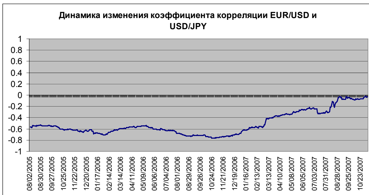
Рис. 38. График динамики изменения коэффициента корреляции , рассчитанный по дневным логарифмическим доходностям курсов валют EUR/USD и USD/JPY с временным интервалом 6 месяцев с шагом 1 день. Взаимосвязь уменьшилась.
