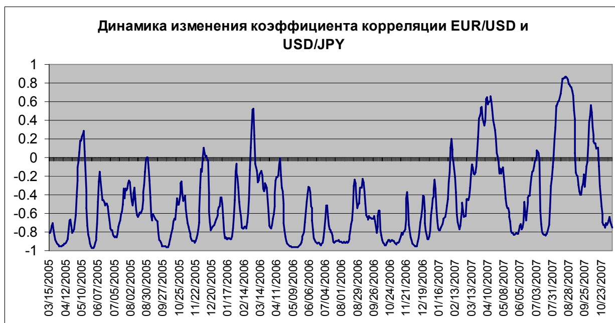
Рис. 18. График динамики изменения коэффициента корреляции по дневным ценам закрытия курсов валют EUR/USD и USD/JPY с временным интервалом 1 месяц с шагом 1 день. Ситуация аналогична предыдущему графику.
