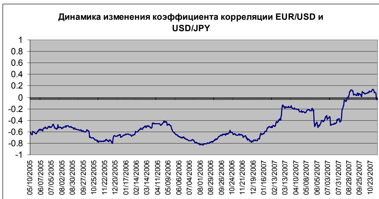
Рис. 37. График динамики изменения коэффициента корреляции , рассчитанный по дневным логарифмическим доходностям курсов валют EUR/USD и USD/JPY с временным интервалом 3 месяца с шагом 1 день. В 2007 году взаимосвязь данных валют начала изменяться, и перестала быть такой сильной, как до 2007 года.
