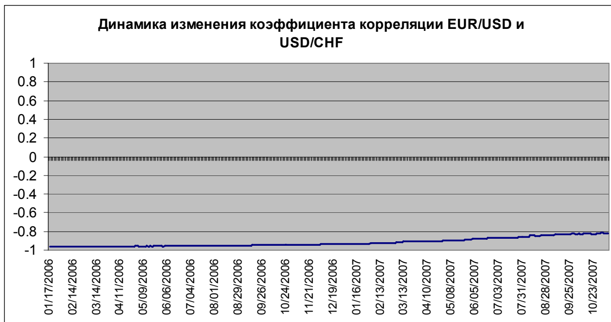
Рис. 33. График динамики изменения коэффициента , рассчитанный по дневным логарифмическим доходностям курсов валют EUR/USD и USD/CHF с временным интервалом 1 год с шагом 1 день. Валюты показывают сильную отрицательную взаимосвязь (при росте одной валюты другая падает).
